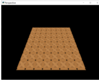
Fig. 101: perspective
