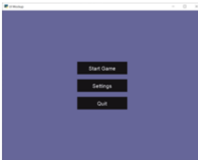
Fig. 80: gui_flat_button
